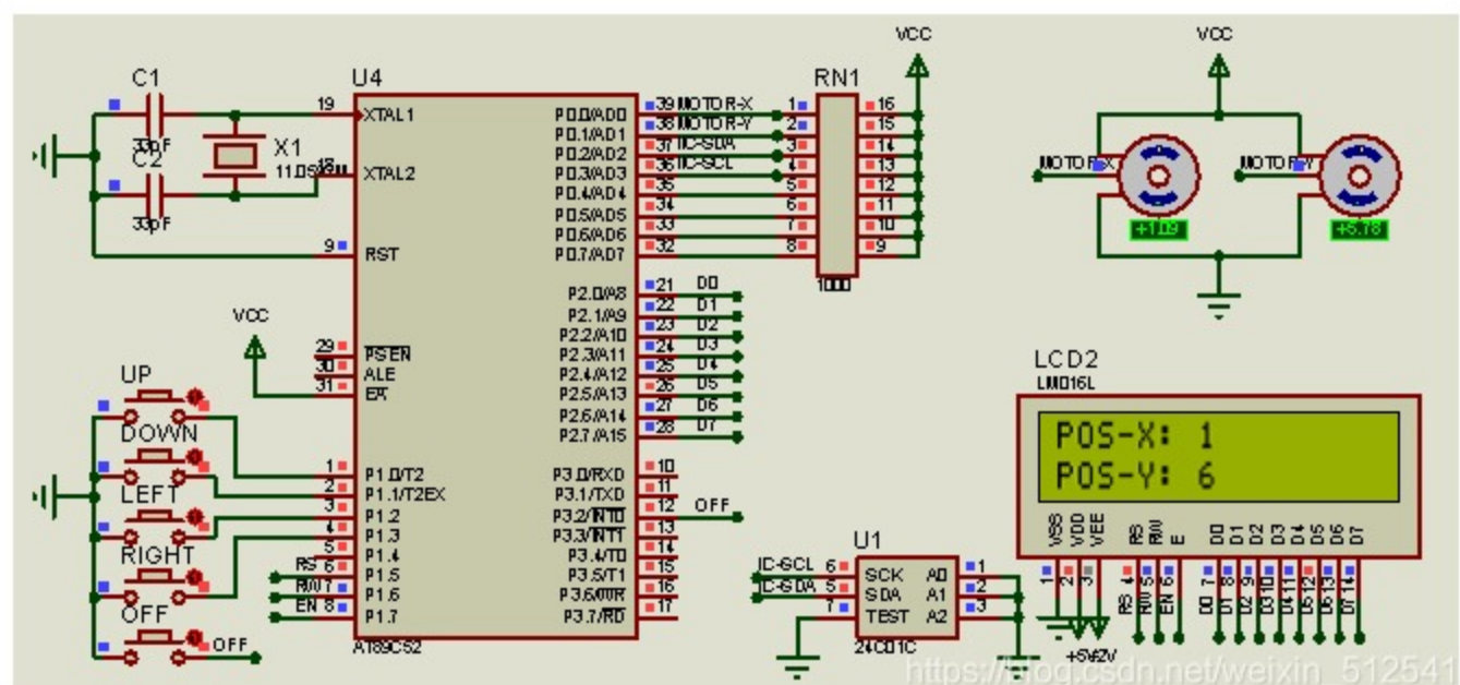
MCU控制器电路
